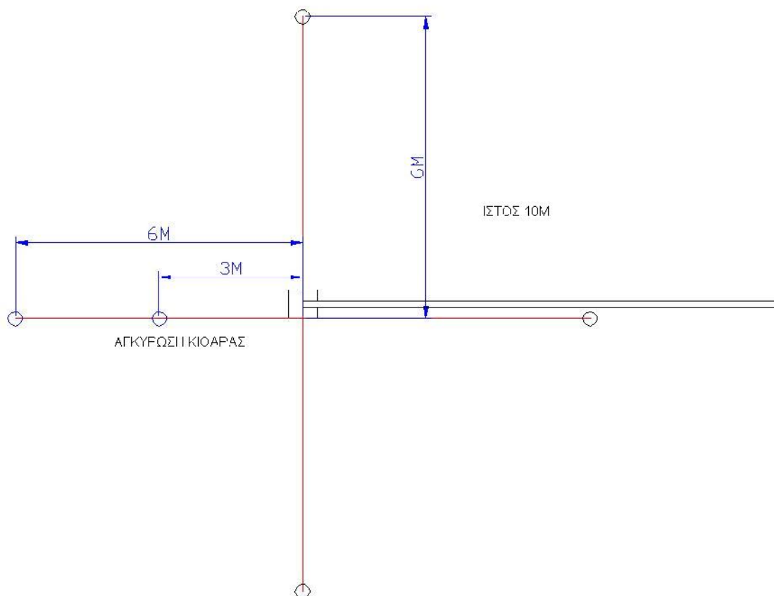
1. Εικόνα Διάγραμμα αγκυρώσεων Ιστού 10μ
